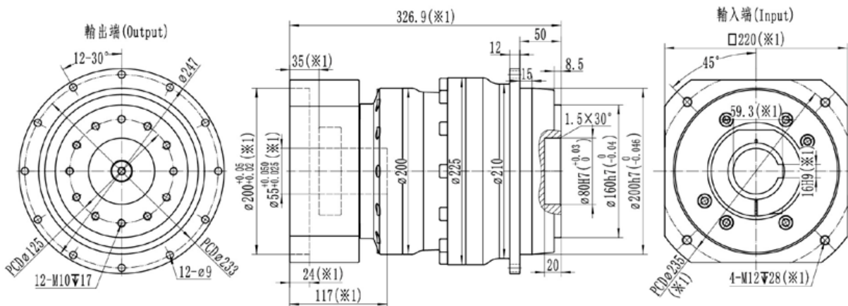
最大55(※2)夾緊孔直徑
