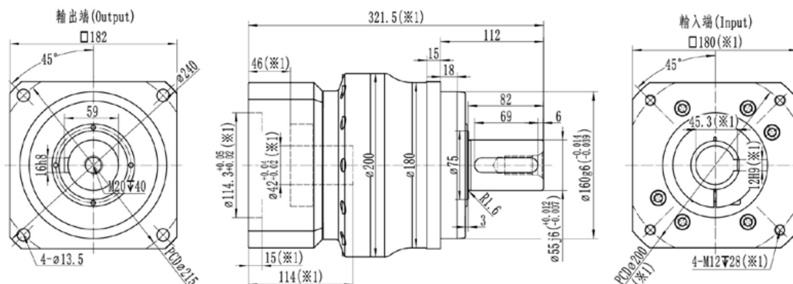
最大55(※2)夾緊孔直徑
